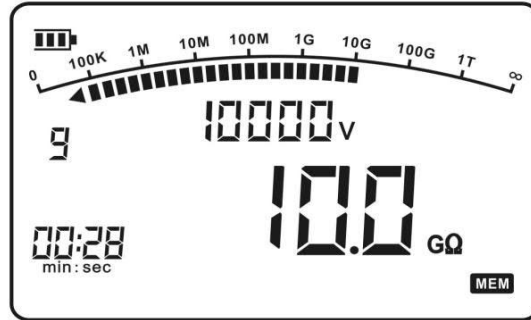
图5：查询状态显示
