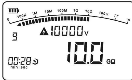
图4：测试状态液晶显示界面
