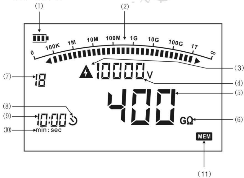
图2: BC2303液晶显示内容
