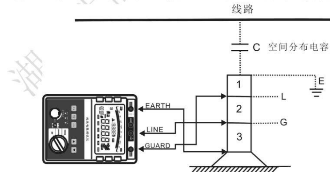
图6：利用屏蔽端（GUARD）屏蔽干扰 其它方面的应用可参考此接法。
